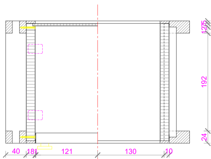
C-C
