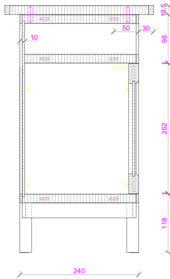
B-B
